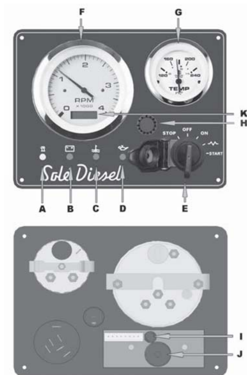
Стандартная панель управления, 12 В
