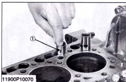
(1) Толкатель
