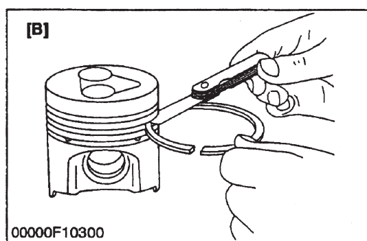
(В) Второе компрессионное кольцо и маслосъемное кольцо
