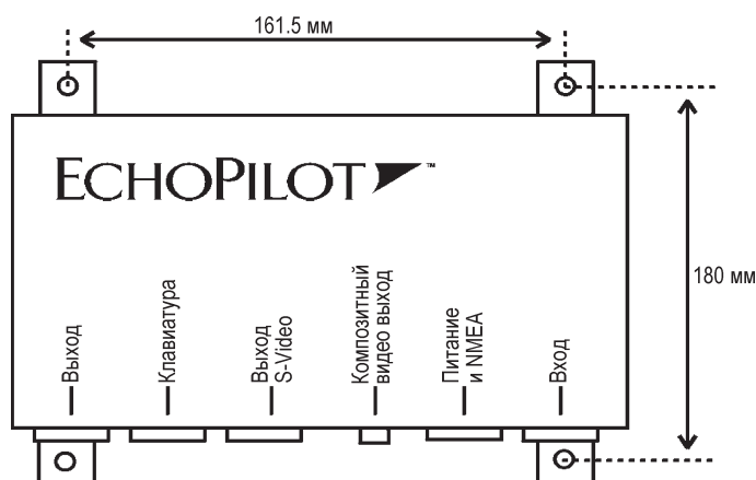
Монтажные размеры интерфейсного видеоблока
