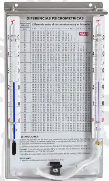
25.0635 Psicrómetro Psychrometer Psychromètre 215x120 mm
